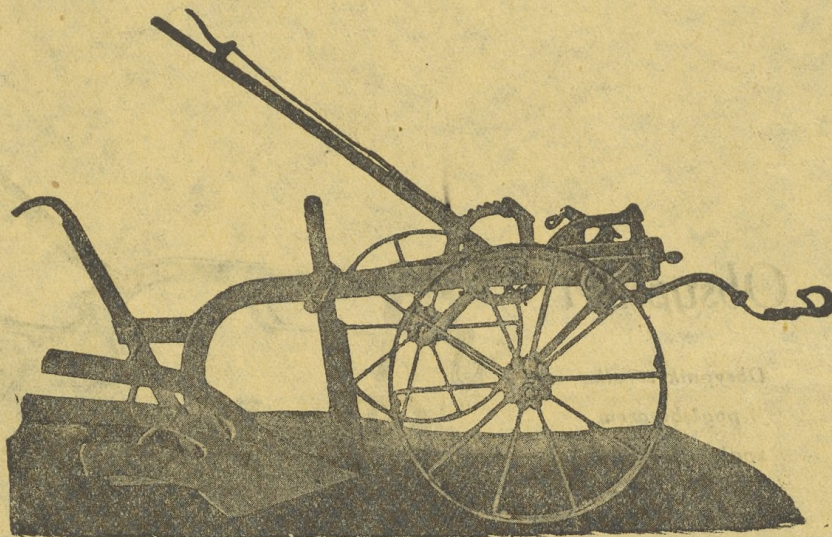
Pług „Zwycięzca“ TRSA z ażurową odkładnią na gleby lepkie
