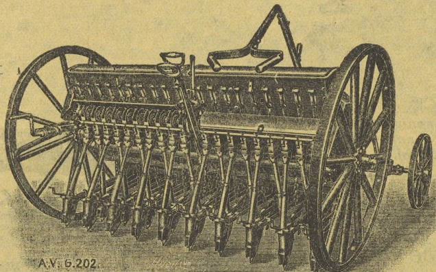
Siewnik normalny „trybikowy”.
