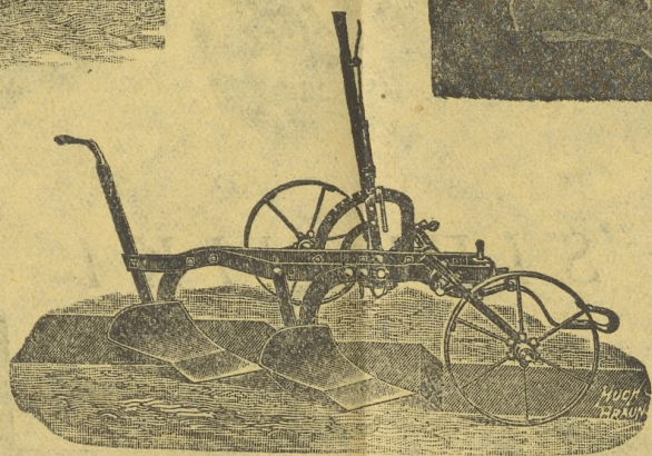
Pług 2-skibowy „Correct“ w normalnem wykonaniu. Użycie wielostronne z najrozmaitszymi dodatkami.
